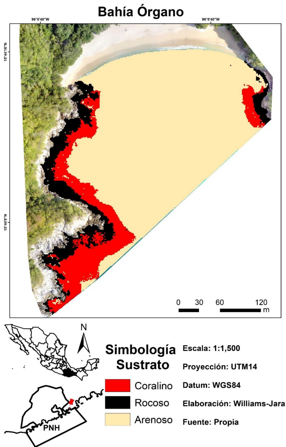
Figura 29. Mapa temático de Bahía Órgano.
