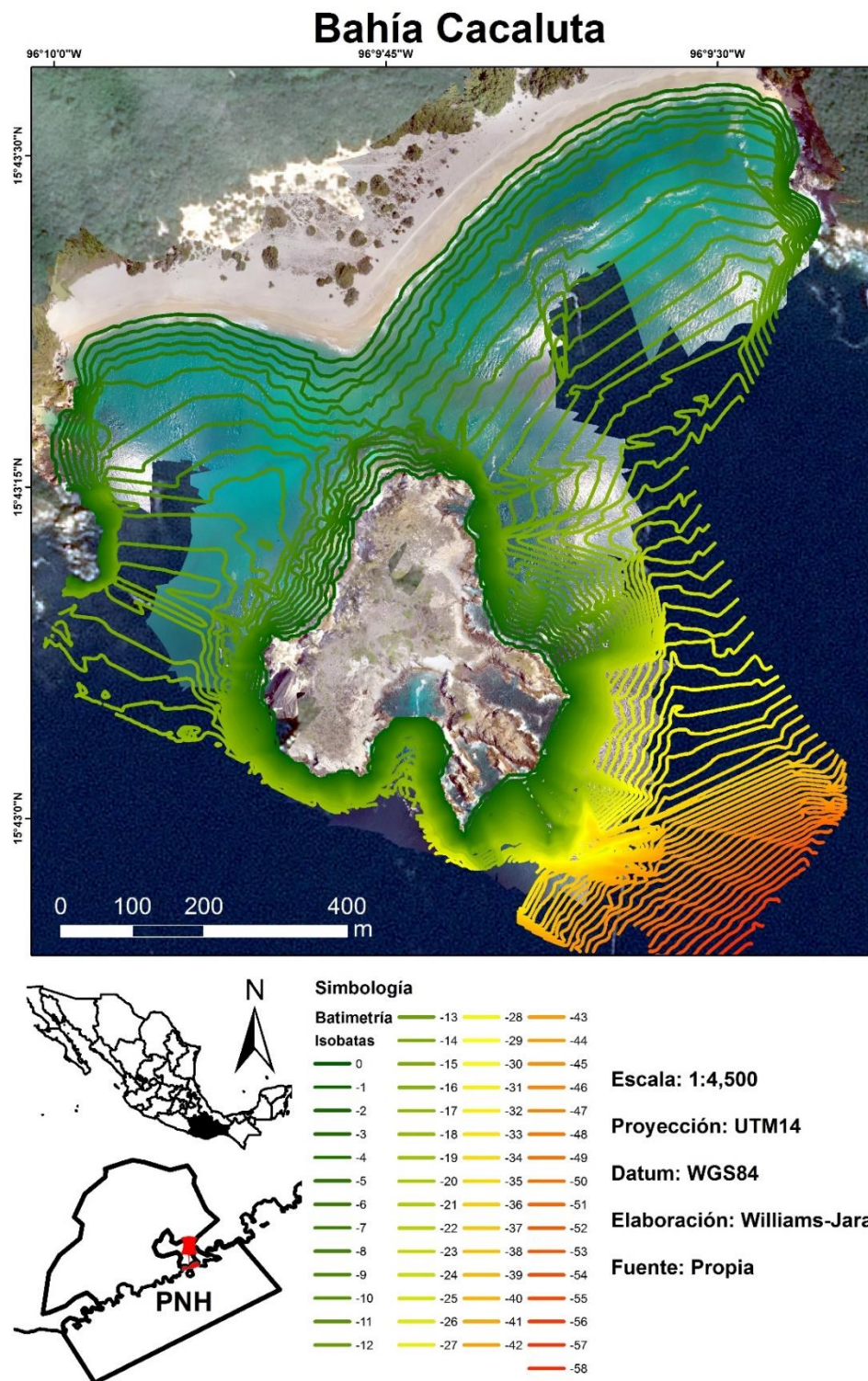
Figura 33. Mapa isobático de Bahía Cacaluta (Imagen SPOT 5 de fondo, generado con datos provenientes de la “ERMEXNG-ermex0169, 2017).
