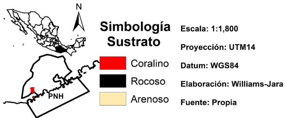
Figura 25. Mapa temático de Bahía Riscalillo.
