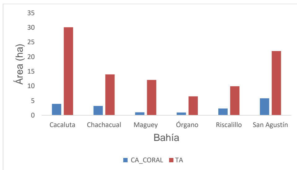
Figura 11. Comparación entre el área total (TA) de las bahías del PNH y su cobertura de coral, estimadas a partir de las ortofotos.
