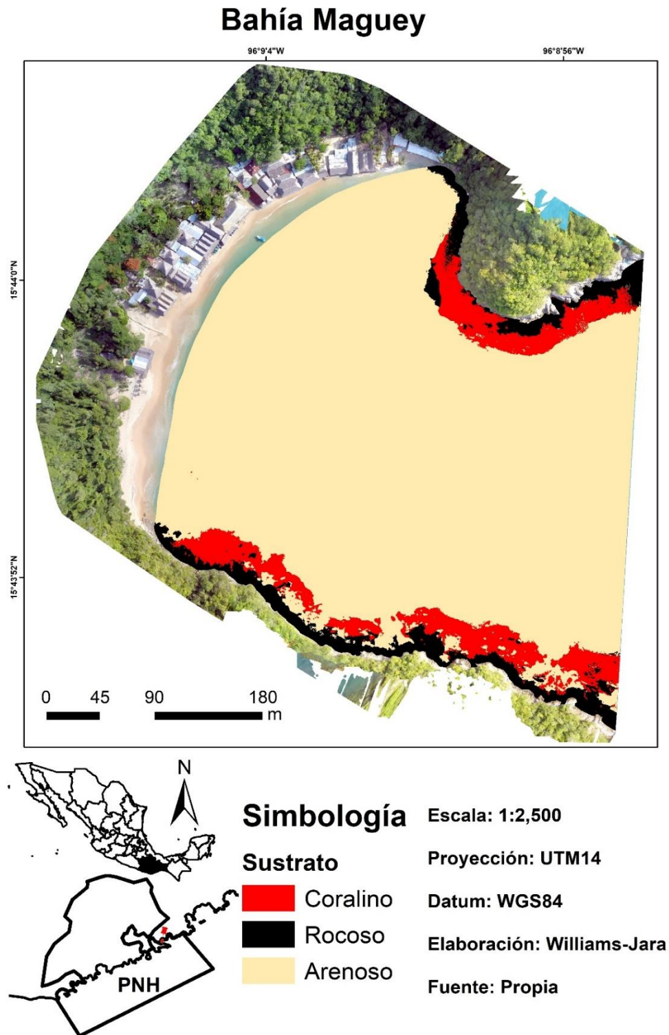
Figura 28. Mapa temático de Bahía Maguey.
