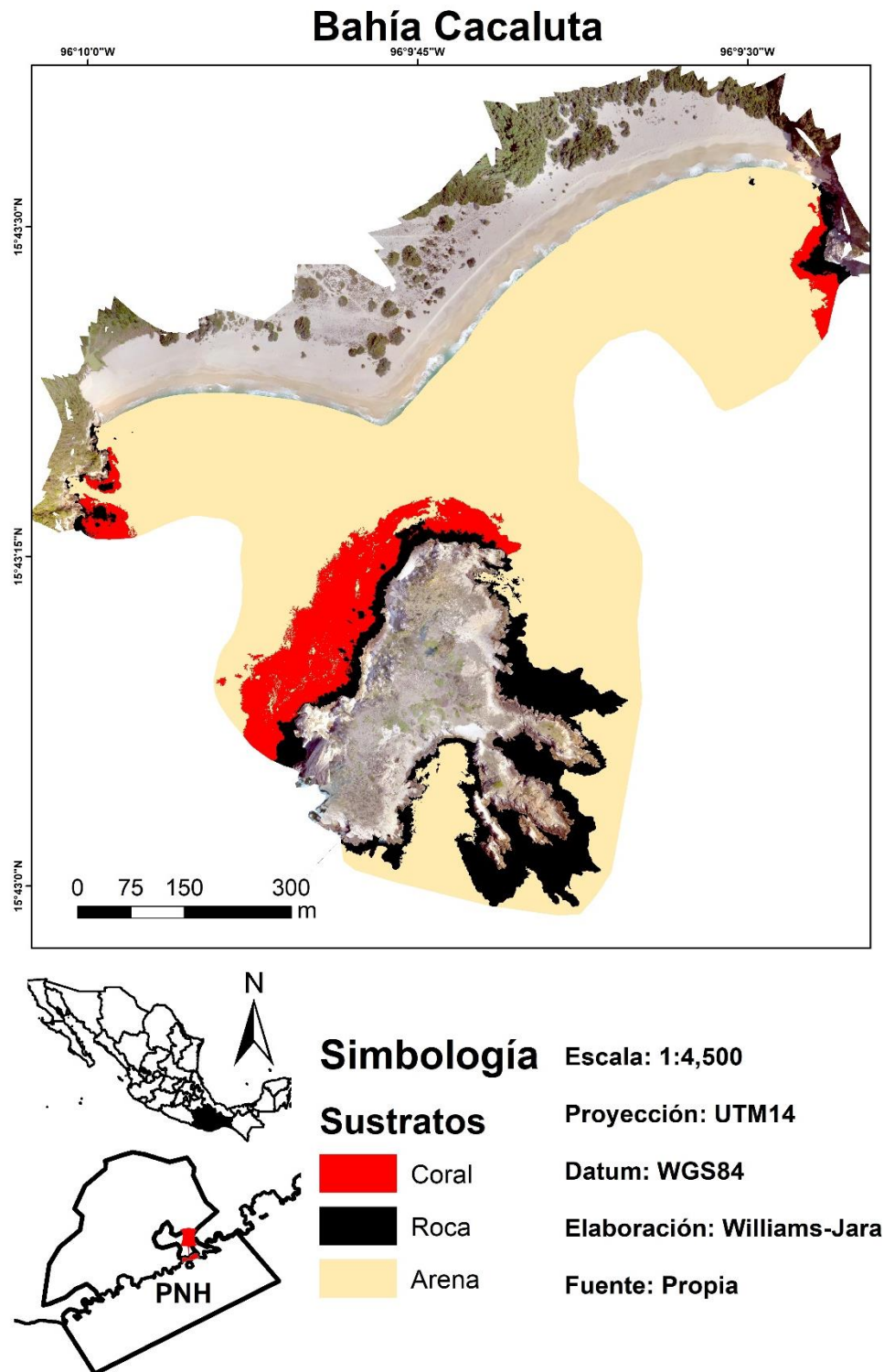
Figura 27. Mapa temático de Bahía Cacaluta.
