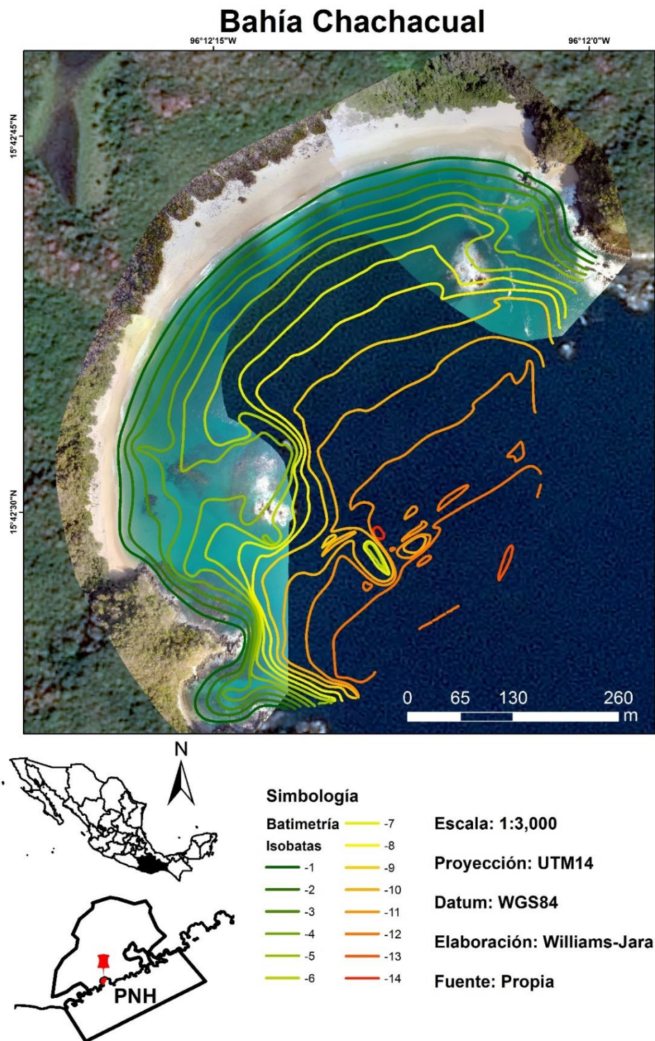
Figura 31. Mapa isobático de Bahía Chachacual (Imagen SPOT 5 de fondo, generado con datos provenientes de la “ERMEXNG-ermex0169, 2017).
