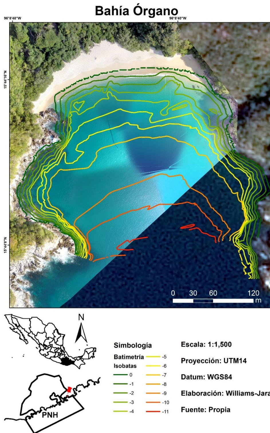
Figura 35. Mapa isobático de Bahía Órgano (Imagen SPOT 5 de fondo, generado con datos provenientes de la “ERMEXNG-ermex0169, 2017).
