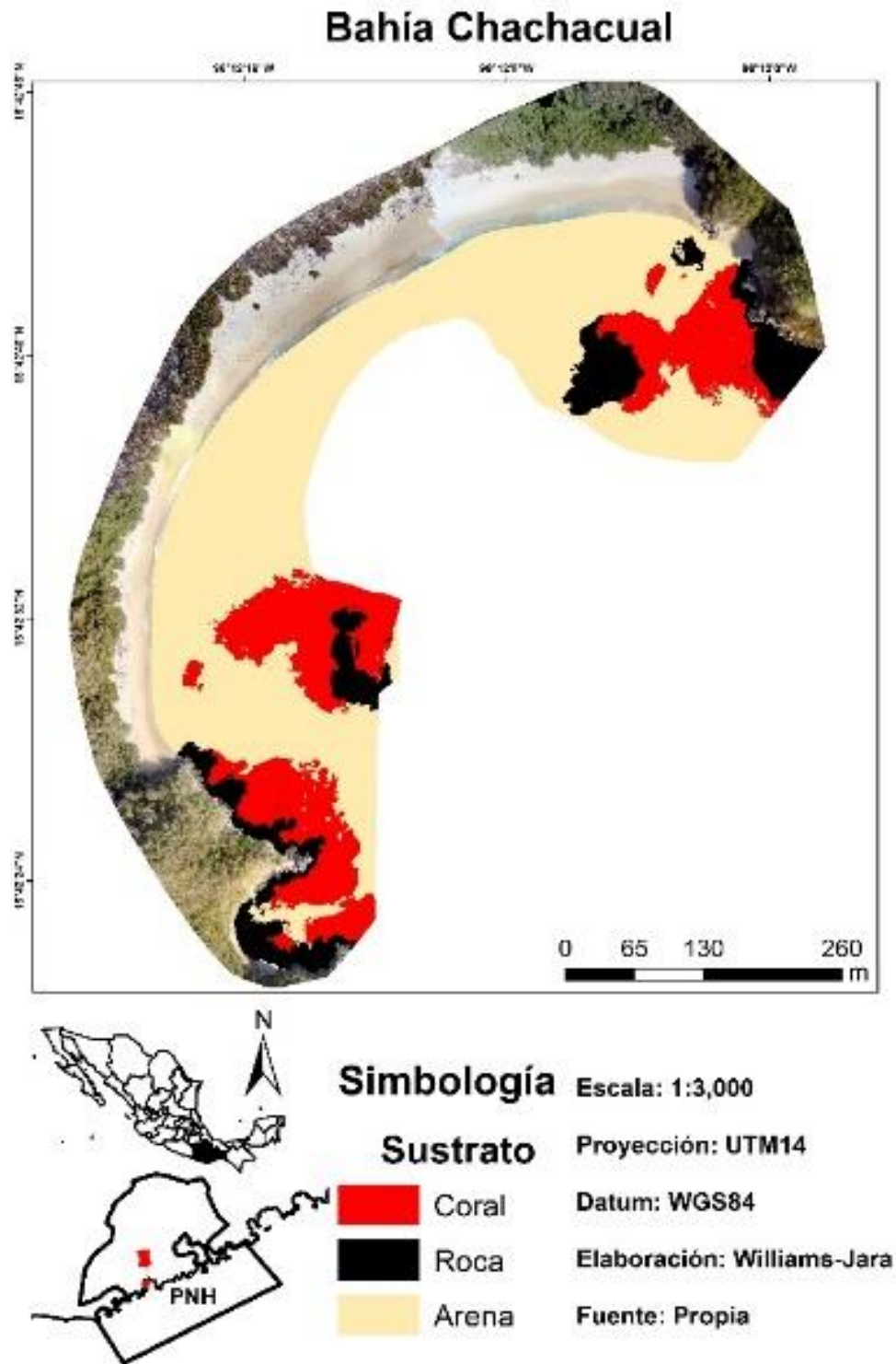
Figura 26. Mapa temático de Bahía Chachacual.
