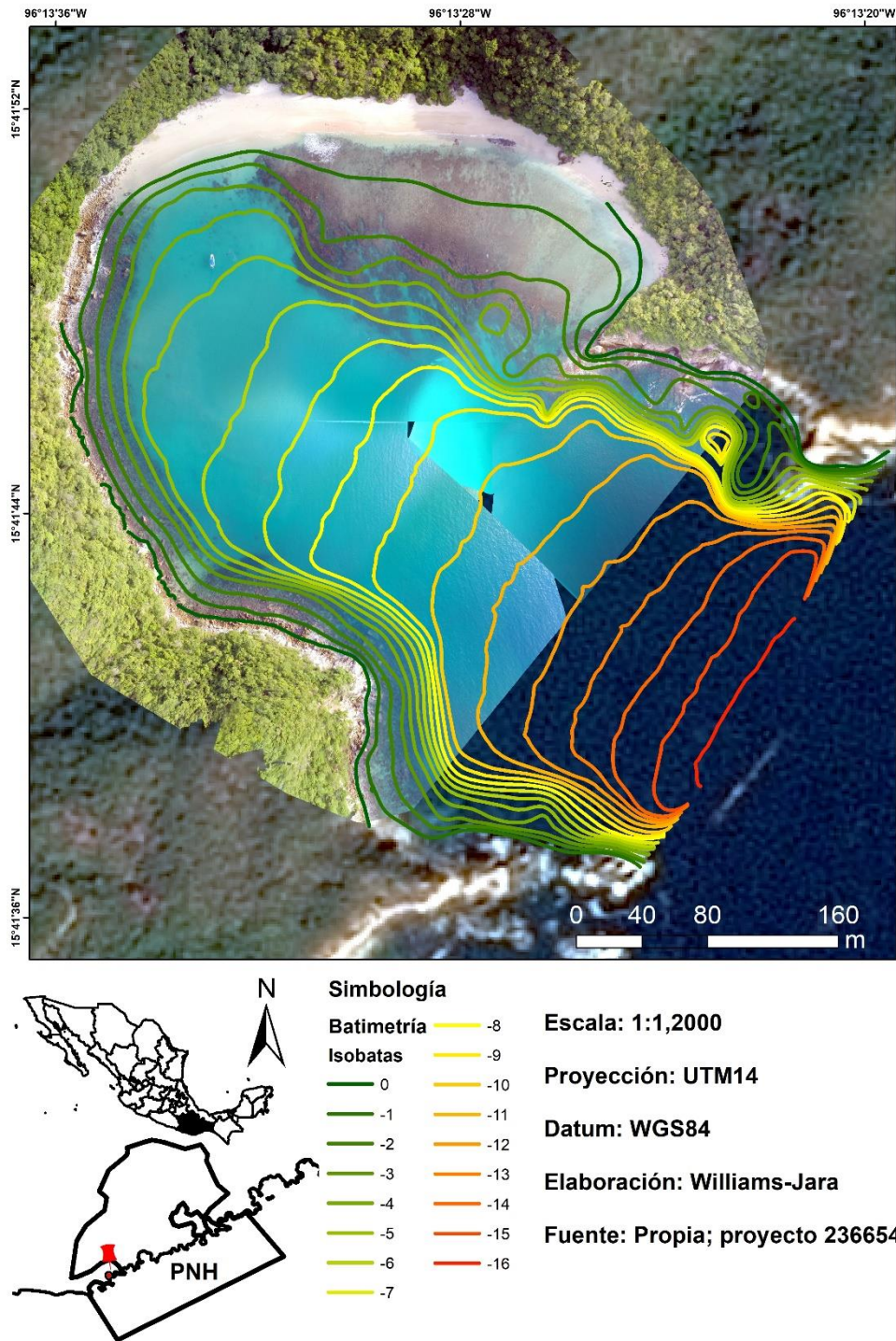
Figura 32. Mapa isobático de Bahía Riscalillo (Imagen SPOT 5 de fondo, generado con datos provenientes de la “ERMEXNG-ermex0169, 2017).
