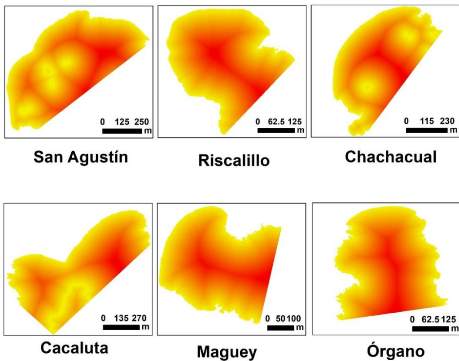
Figura 16. Mapa de distancias (en metros), donde el rojo corresponde a los sitios más alejados de la línea de costa y el amarillo a los más cercanos a esta.
