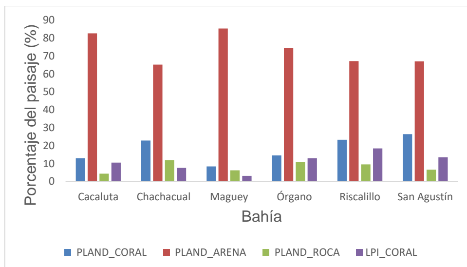
Figura 12. Comparación del porcentaje de cada tipo de sustrato en el paisaje (PLAND), así como el porcentaje del paisaje que ocupa el parche más grande de coral (LPI).
