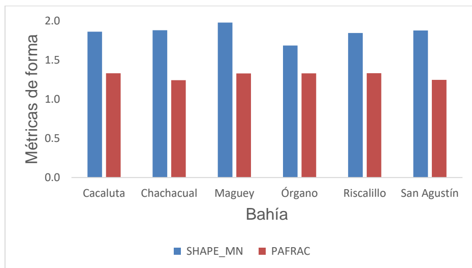
Figura 14. Métricas que indican la complejidad de la forma para la clase coral por bahía.
